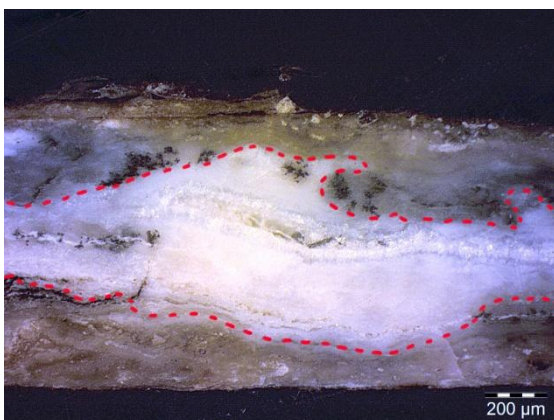
Figure 75 : Localisation de CP3.CP1i, 1008-1a, MO, DF, 50x ©HECR-Arc, 2013.
