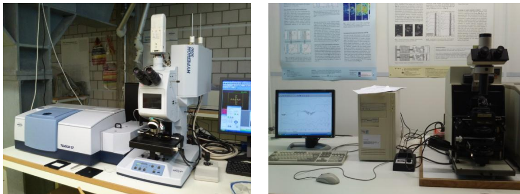
Figure 20 : Vue des appareils utilisés pour l'analyse FTIR : Bruker® Hyperion 3000 (à gauche) et Perkin® Elmer System 2000 (à droite) ©HECR-Arc, 2013.
