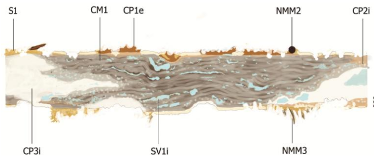
Figure 93 : Stratigraphie de la plaque 1010-28 nettoyée ©HECR-Arc, 2013.
