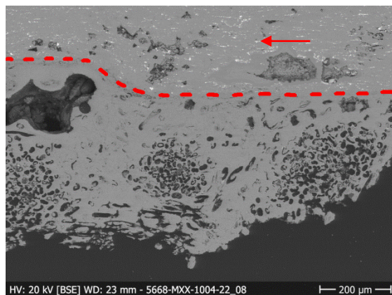
Figure 105 : Localisation de la limite grâce à la présence du plomb dans la strate de corrosion CM1 (B), image SEM, BSE, 1004-22 ©IMA, 2013.
