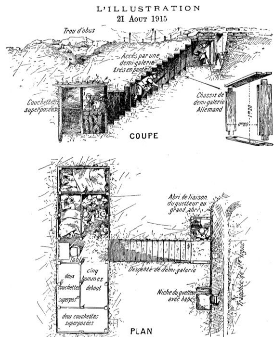
Type d'abri allemand en première ligne, avec accès par une demi-galerie en escalier.
