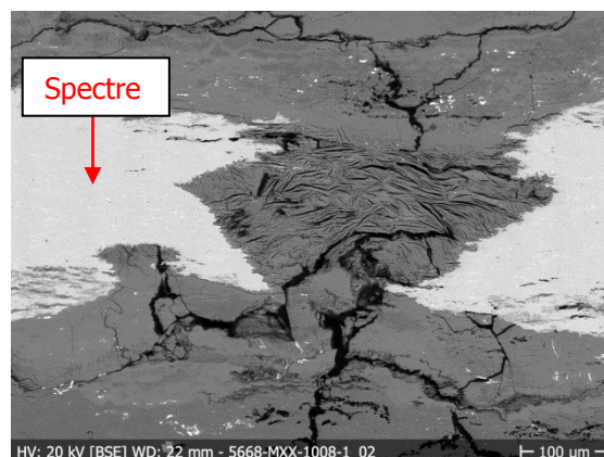
Figure 46 : Image SEM, BSE, 1008-1a détail, localisation du spectre* EDS ©IMA, 2013.
