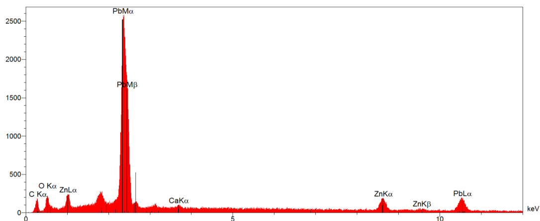
Figure 81 : Spectre d'analyse EDS des inclusions métalliques ©IMA, 2013.
