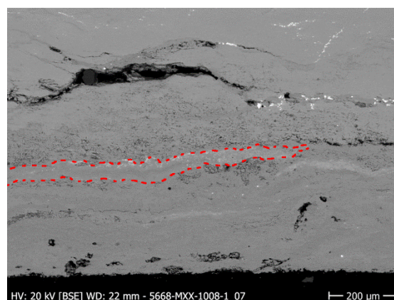
Figure 78 : Absence de métal dans CP4i, image SEM, BSE, 1008-1a ©IMA, 2013.
