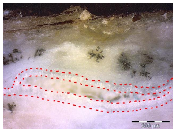
Figure 76 : Localisation de CP3.CP2i, 1008-1a, MO, DF, 50x ©HECR-Arc, 2013.
