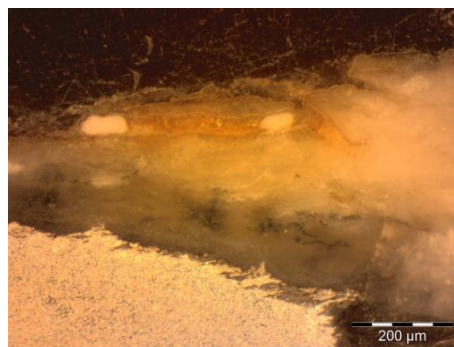
Figure 114 : Interface avant/après le test, 1008-1b, MO, BF, 200x ©HECR-Arc, 2013.
