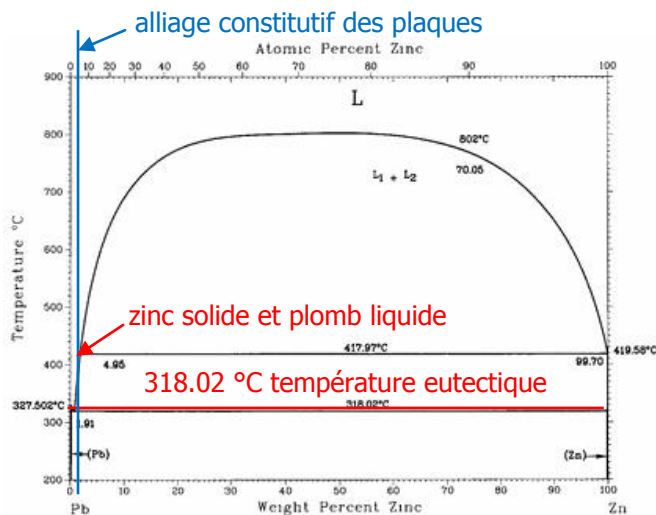
Figure 49 : Diagramme de phase de l'alliage binaire ZnPb © Moser, et al., 1994.
