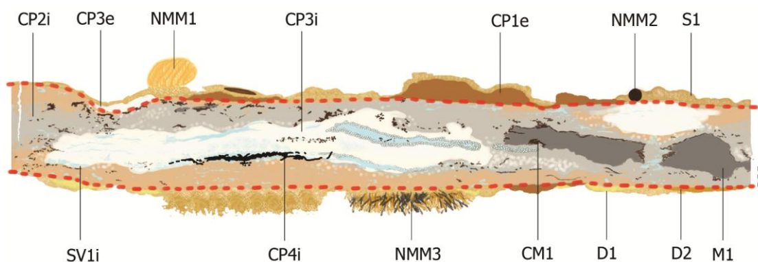
Figure 101 : Localisation de la limite de la surface d'origine (en rouge) sur la stratigraphie comportant CP2i comme couche de corrosion principale ©HECR-Arc, 2013.
