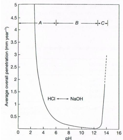
Figure 94 : Effet du pH sur la vitesse de corrosion du zinc (milieu aqueux). A et C : corrosion rapide, B : corrosion lente (film stable) ©Goodwin, 2010.
