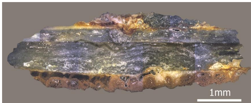
Figure 42 : Coupe transversale échantillon 1004-22, MO, DF, 50x ©HECR-Arc, 2013.
