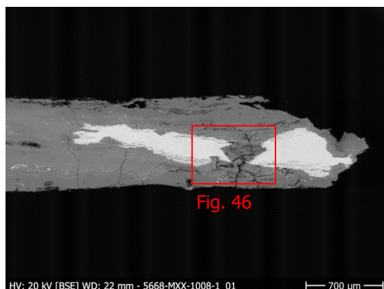
Figure 45 : Image SEM, BSE, 1008-1a, localisation de la Fig. 46 ©IMA, 2013.
