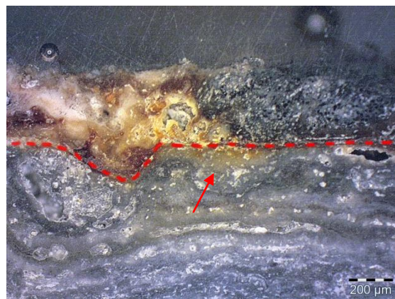
Figure 106 : Localisation de la limite et présence de produits de corrosion dans la strate CM1 (B), 1004-22, MO, DF, 50x ©HECR-Arc, 2013.
