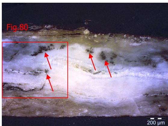
Figure 79 : Localisation des inclusions CM1 (A) en feuillets et de la Fig. 80, 1008-1a, MO, DF, 50x ©HECR-Arc, 2013.
