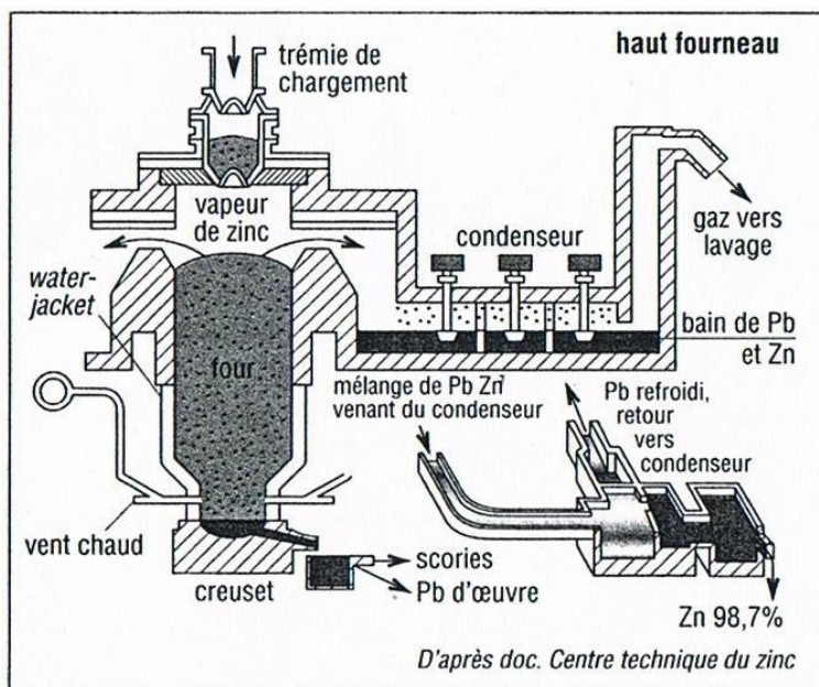
Figure 157 : Procédé « imperial smelting » ©Barralis et Maeder, 2001.
