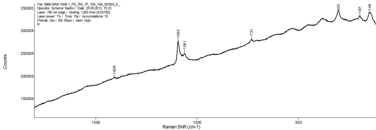
Figure 146 : Spectre Raman, 1008-1a, zone blanche : grande fluorescence, mélange de smithsonite et d'autres produits de corrosion [1410, 1093s, 1061m, 732, 304s, 197m 146s cm-1] ©HKB, 2013.
