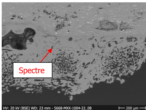
Figure 150 : Localisation du spectre, image SEM, BSE, 1004-22, et spectre d'analyse EDS montrant la présence d'oxygène et de zinc ©IMA, 2013.
