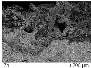
Figure 62 : Répartition du zinc et du soufre, image SEM, BSE, 1004-22 ©IMA, 2013.
