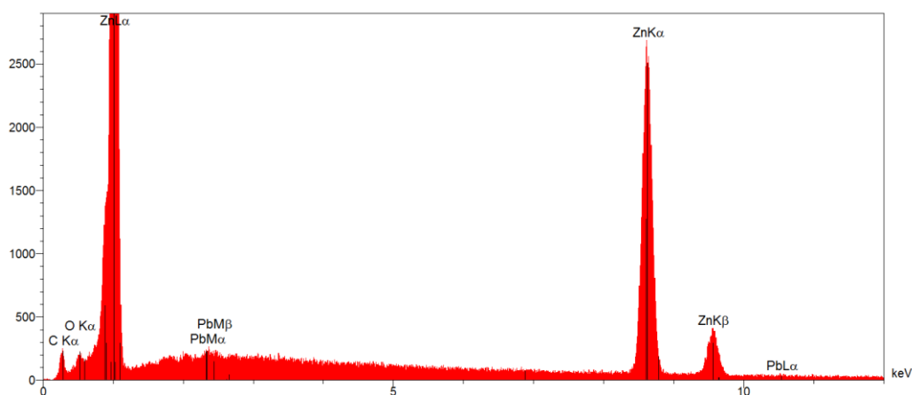
Figure 47 : Spectre d'analyse EDS du noyau métallique restant ©IMA, 2013.
