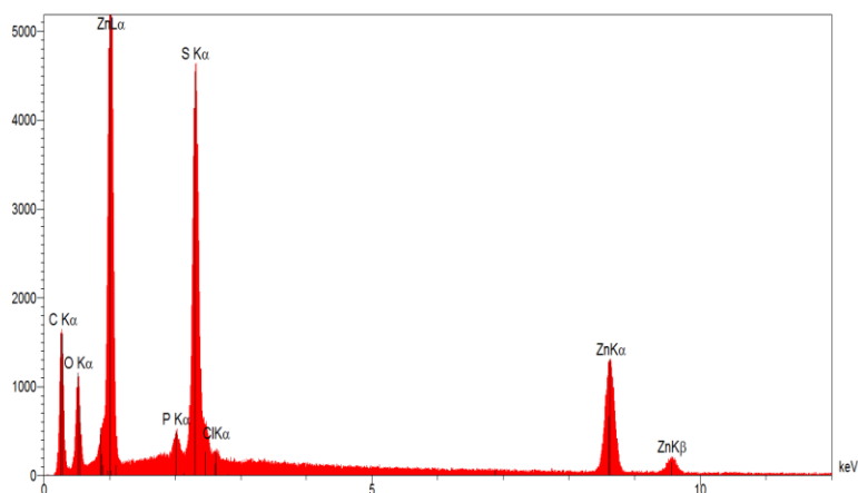
Figure 71 : Spectre d'analyse EDS de la strate mineure CP2.CP2i sur l'échantillon 1008-1a montrant la présence de soufre et de zinc ©IMA, 2013.
