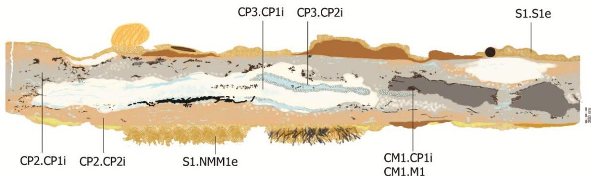
Figure 51 : Stratigraphie représentante la plaque en coupe transversale et les strates mineures
