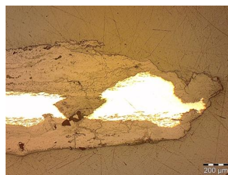
Figure 44 : Mise en évidence du métal non-corrodé (en blanc), 1008-1a, MO, BF, 50x ©HECR-Arc, 2013.
