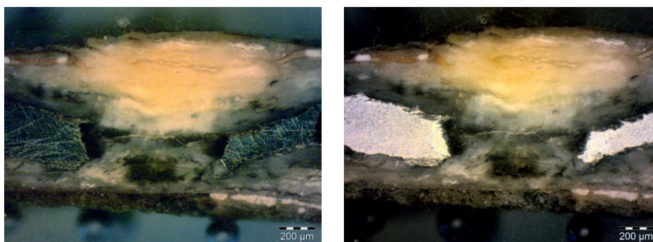
Figure 116 : Echantillon avant/après le test, 1008-1b, MO, DF, 200x ©HECR-Arc, 2013.
