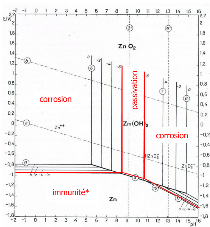
Figure 151 : Diagramme d'équilibre tension-pH du système zinc-eau, à 25°C ©De Zoubov et Pourbaix, 1963.
