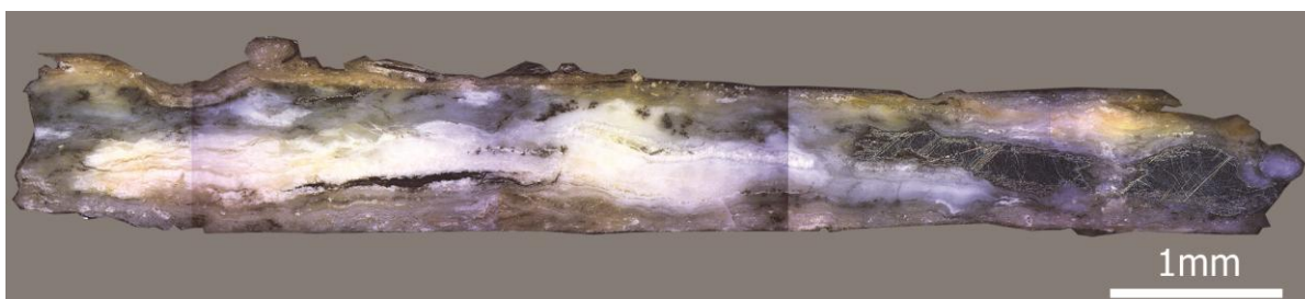
Figure 43 : Coupe transversale échantillon 1008-1, MO, DF, 50x ©HECR-Arc, 2013.
