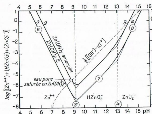
Fig. 4. — Influence du pH sur la solubilité des hydroxydes de zinc, à 25°C.
