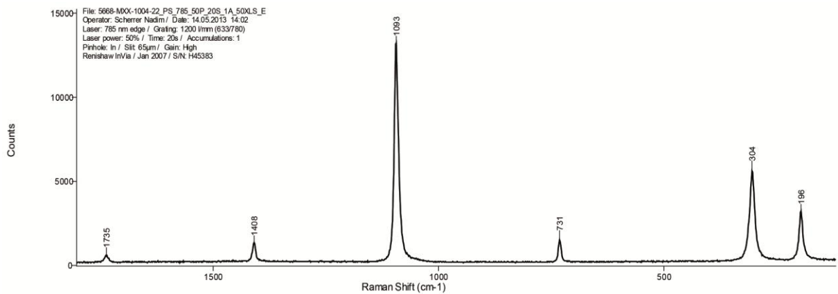
Figure 148 : Spectre Raman, 1004-22, zone grise : smithsonite ( ZnCO_3 , groupe calcite) [1736, 1408, 1092vs, 730, 303s, 196m cm^{-1} ] ©HKB, 2013.
