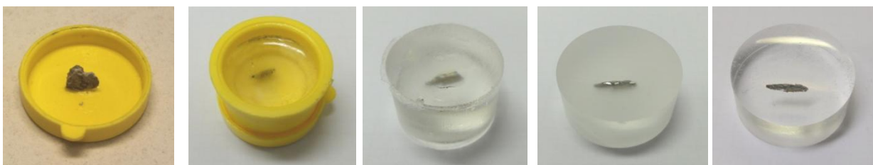
Figure 126 : Etapes de préparation de l'échantillon : positionnement et collage, enrobage de résine, démoulage, polissage à la machine et à la main @HECR-Arc, 2013.
