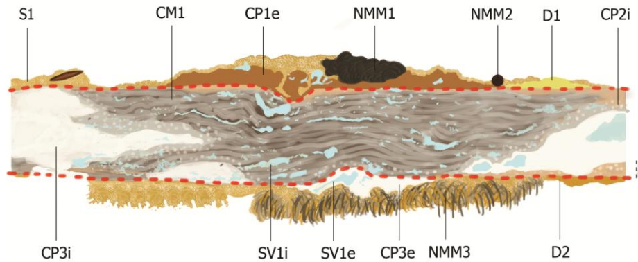
Figure 102 : Localisation de la limite de la surface d'origine (en rouge) sur la stratigraphie comportant CM1 (B) comme couche de corrosion principale ©HECR-Arc, 2013.
