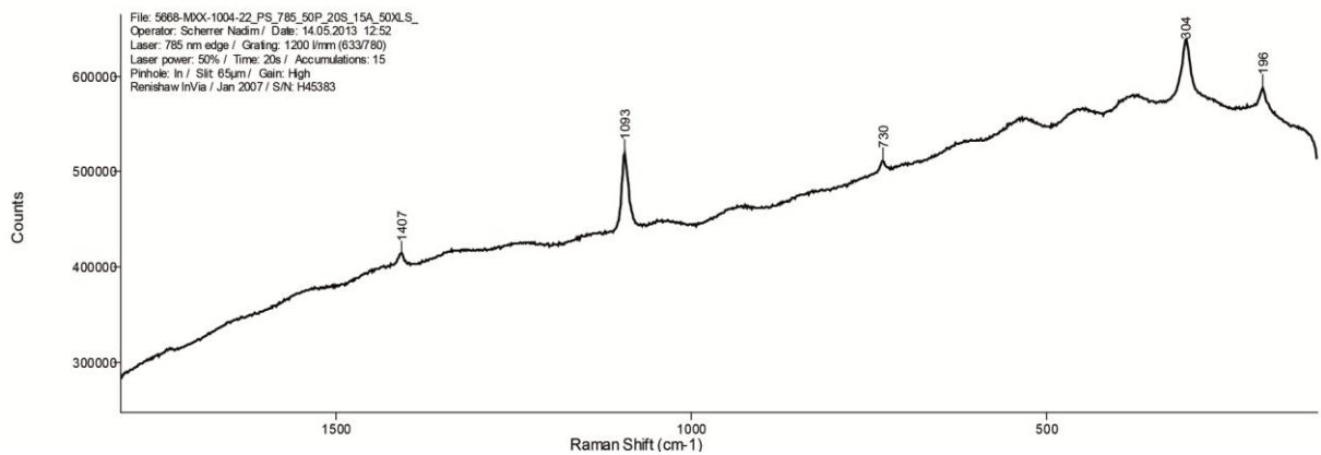
Figure 149 : Spectre Raman, 1004-22, zone blanche : mélange de smithsonite et d'un autre composé non-déterminé due à grande fluorescence [1093vs, 304m cm^{-1} ] ©HKB, 2013.
