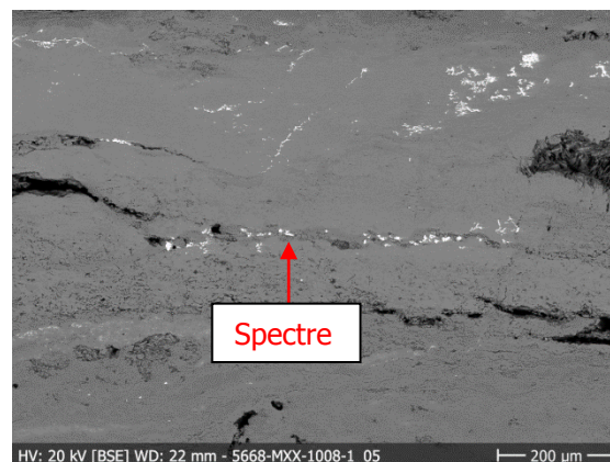
Figure 80 : Inclusions de plomb visibles en blanc, localisation du spectre EDX, image SEM, BSE, 1008-1a ©IMA, 2013.
