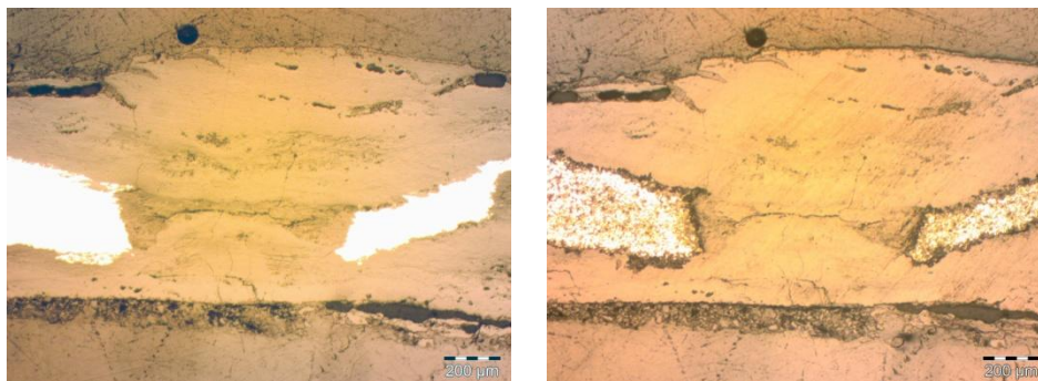
Figure 115 : Echantillon avant/après le test, 1008-1b, MO, BF, 200x ©HECR-Arc, 2013.
