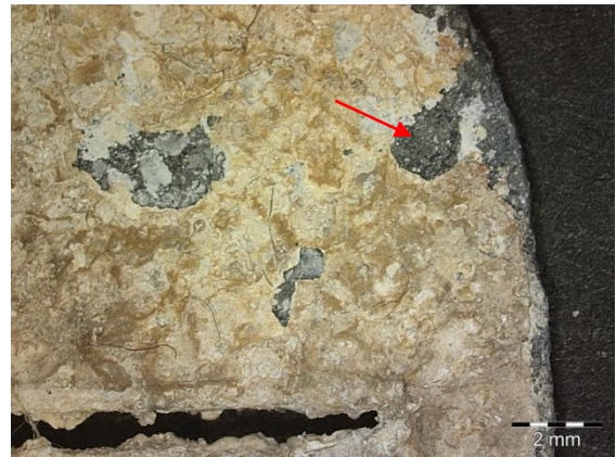
Figure 84 : Vue de CM1 (B) en surface, 1010-28 verso, loupe binoculaire, 0.67x ©HECR-Arc, 2013.
