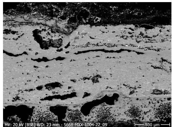
Figure 86 : Inclusions de plomb horizontales (en blanc), image SEM, BSE, 1004-22 ©IMA, 2013.
