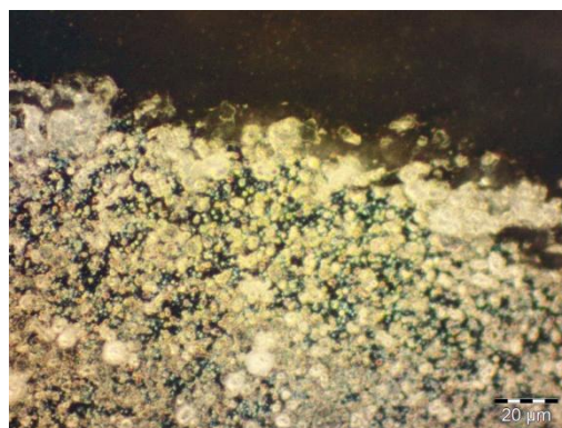
Figure 113 : Aspect de la surface du métal, 1008-1b, MO, DF, 50x ©HECR-Arc, 2013.
