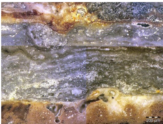
Figure 85 : Structure de la strate en coupe, 1004-22, MO, DF, 50x ©HECR-Arc, 2013.
