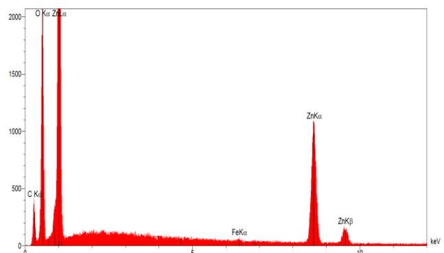
Figure 150 : Localisation du spectre, image SEM, BSE, 1004-22, et spectre d'analyse EDS montrant la présence d'oxygène et de zinc ©IMA, 2013.
