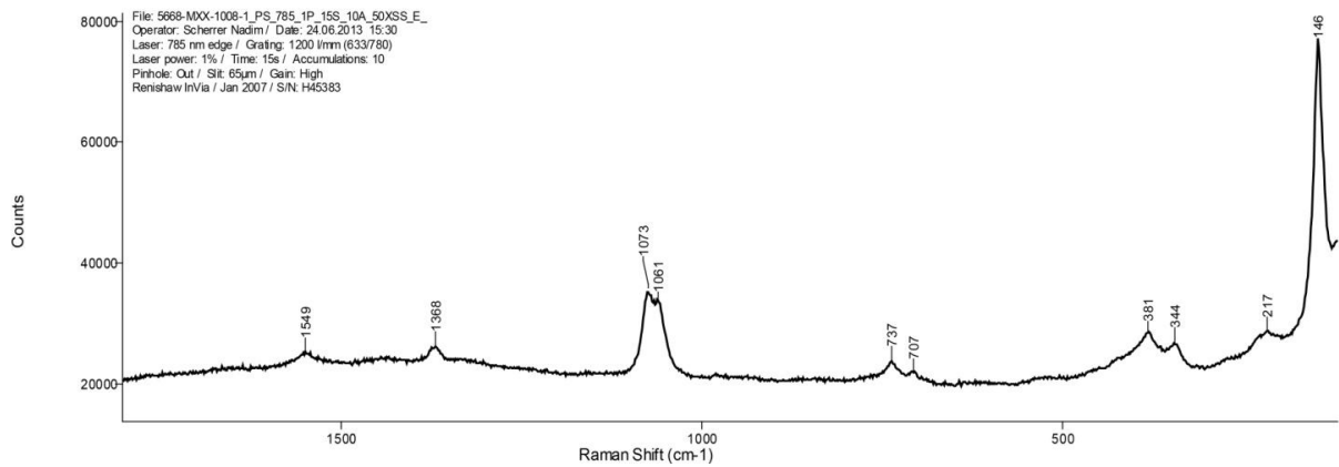
Figure 145 : Spectre Raman, 1008-1a, zone grise à gris-orange: non-déterminé [1550, 1370, 1076s, 1059s, 737, 705, 382, 343, 220, 147vs cm-1] ©HKB, 2013.
