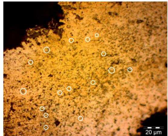
Figure 50 : Nodules de plomb détectés (en blanc), 1008-1b, attaqué par HCl 10%, MO, BF, 500x ©HECR-Arc, 2013.
