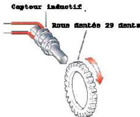
Figure 16 : Capteur de vitesse et roue dentée
